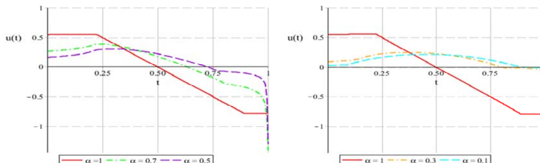
شکل ۲،۴. نمودارهای تقریبی تابع کنترل u(t) برای مثال ۱،۴ به ازای N = 4 و M = 6 برای \alpha = 1, 0.7, 0.5 (سمت چپ) و \alpha = 1, 0.3, 0.1 (سمت راست).
